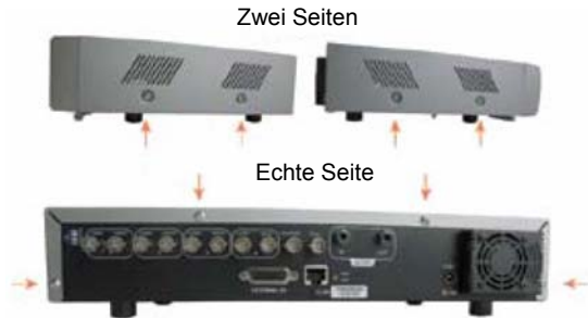
Schritt 1-1: Entfernen Sie die Schrauben
