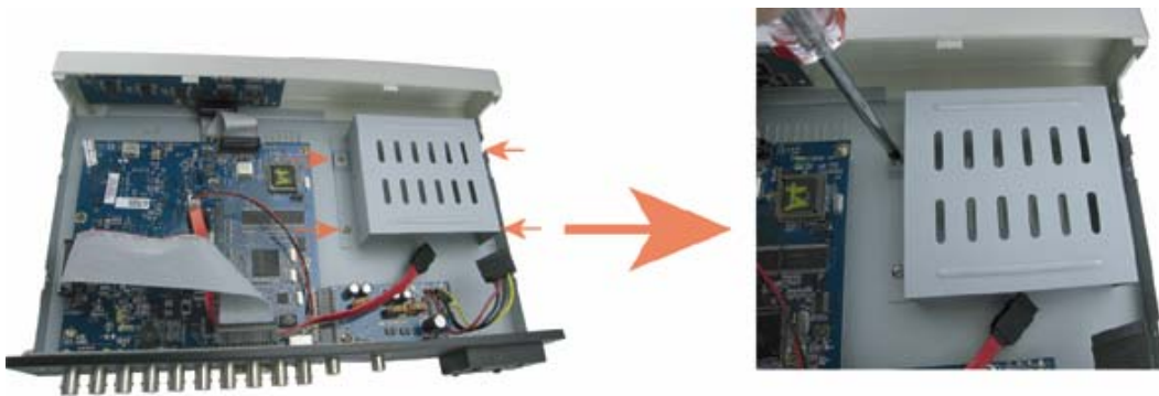
Schritt 2: Entfernen Sie die HDD-Halterung.
